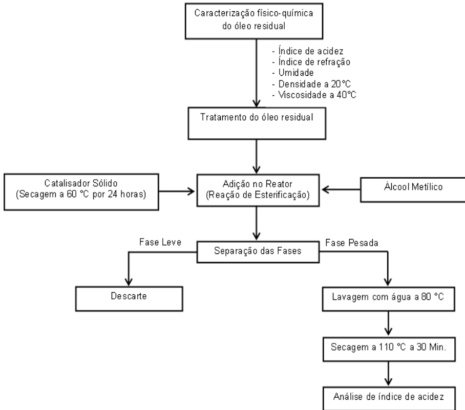
Figura 1. Fluxograma da caracterização físico-química e do processo do tratamento do óleo residual
