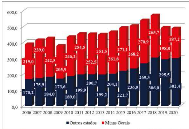
Gráfico 1 – Evolução da matriz ferroviária no transporte de cargas: participação do estado de Minas Gerais (1.000.000 de toneladas)
