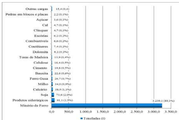
Gráfico 2 – Minas Gerais: produtos transportados em ferrovias, acumulado no período de 2006 a 2020 (Quantidades em 1.000.000 de toneladas e percentuais)
