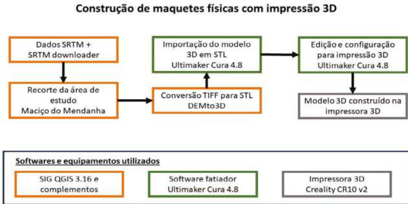
Figura 9 – Etapas para a construção da maquete por impressão 3D
